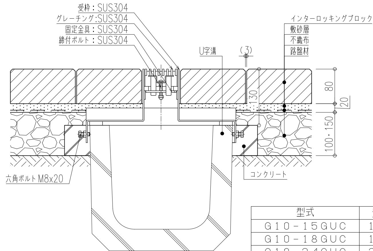
施工参考図
